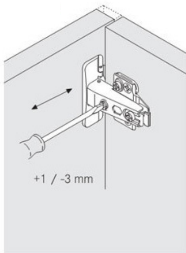
Réglage vertical
