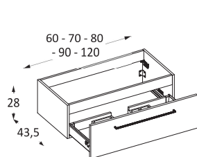
1 tiroir
