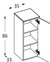
Demi colonne
