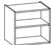
Niche basse H 56 L 60 > L 60 x P 45,5 x H 56 cm
