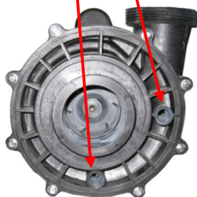
5.1 Positionnement des bouchons sur les pompes 1 et 2
